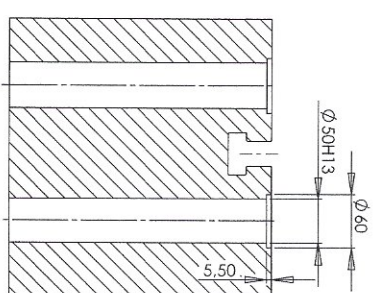
SECTION A-A SCALE 1 : 4
